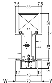
B方立
