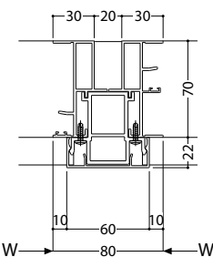
KA方立
