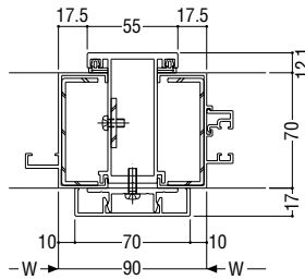
A方立
