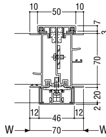
A方立
