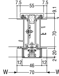
A 1 方立
