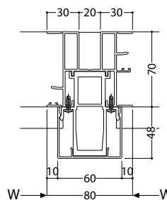
KB方立
