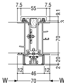
A1方立
