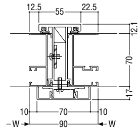
A1方立
