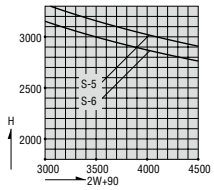
B方立
