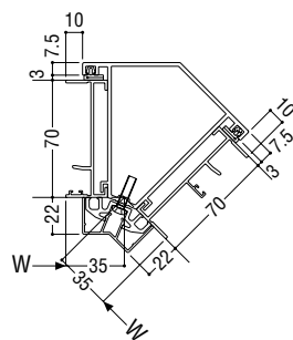
出隅 (135°)
