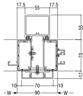
B方立
