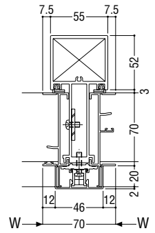
B方立
