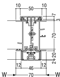
A方立
